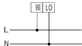
交流电压(≤660V时)直接接入
