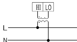
交流电压(>660V时)互感器接入
