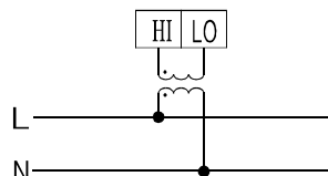
交流电压(>660V时)互感器接入
